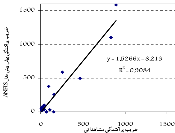
شکل ۵- مقایسه نتایج مدل ANFIS با داده‌های واقعی در مرحله ارزیابی مدل
