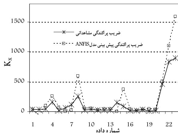
شکل ۶- عملکرد مدل فازی- عصبی در مرحله ارزیابی مدل
