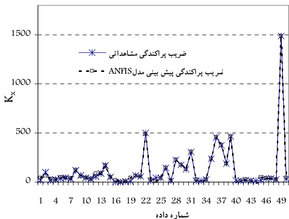
شکل ۴- عملکرد مدل فازی- عصبی در مرحله آموزش مدل
