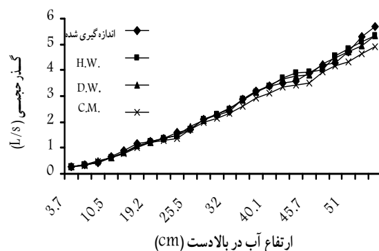
شکل ۷- مقادیر حجمی مشاهده شده و محاسبه شده بر حسب مقادیر مختلف ارتفاع آب بالا دست و برای معادلات مختلف مقاومت برای مدل توپوی ۷/۵ سانتی متری (H.W.: هیزن- ویلیام، D.W.: دارسی- وایسباخ، C.M.: شزی- مانینگ)
