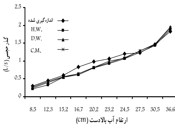
شکل ۸- مقادیر گذر حجمی مشاهده شده و محاسبه شده بر حسب مقادیر مختلف ارتفاع آب بالا دست و برای معادلات مختلف مقاومت برای مدل توپوی ۳/۷ سانتی متری (H.W.: هیزن- ویلیام، D.W.: دارسی- وایسباخ، C.M.: شزی- مانینگ)
