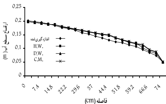
شکل ۱۰- پروفیل سطح آب در مدل توپوی ۷/۵ سانتی متری برای تراز آب بالادست معادل ۵۲ سانتی متر (H.W.: هیزن- ویلیام، D.W.: دارسی- وایسباخ، C.M.: شزی- مانینگ)
