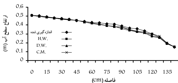
شکل ۹- پروفیل سطح آب در مدل توپوی ۳/۷ سانتی متری برای تراز آب بالادست معادل ۲۰/۲ سانتی متری (H.W.: هیزن- ویلیام، D.W.: دارسی- وایسباخ، C.M.: شزی- مانینگ)
