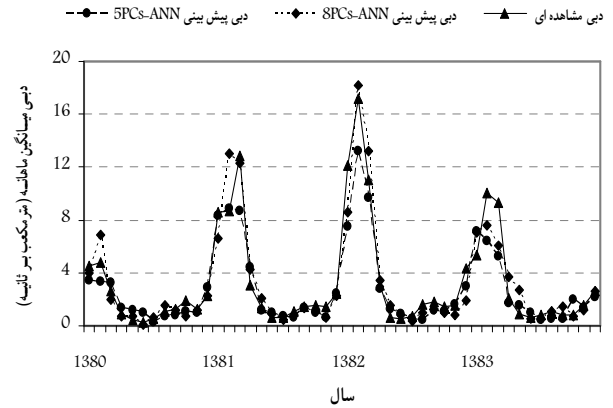
شکل ۸- سری زمانی داده‌های مشاهده‌ای و پیش‌بینی شده برای مدل‌های 5PCs-ANN و 8PCs-ANN در مرحله تست
