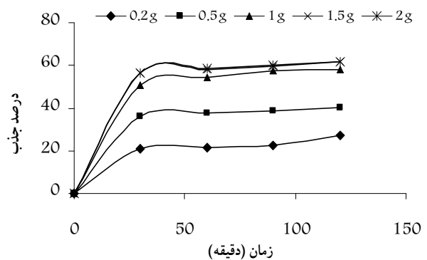
شکل ۳- اثر مقدار جاذب بر درصد جذب مس
