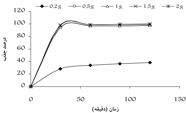
شکل ۵- اثر مقدار جاذب بر درصد جذب آهن
