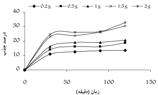
شکل ۴- اثر مقدار جاذب بر درصد جذب سرب
