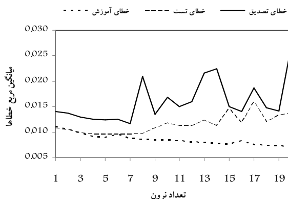
شکل ۶- تغییرات خطای داده‌های آموزش، تست و تصدیق با افزایش تعداد نرون‌های لایه مخفی
