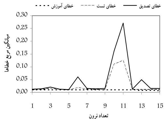
شکل ۴- تغییرات خطای داده‌های آموزش و تست و تصدیق با افزایش تعداد نرون‌های لایه مخفی
