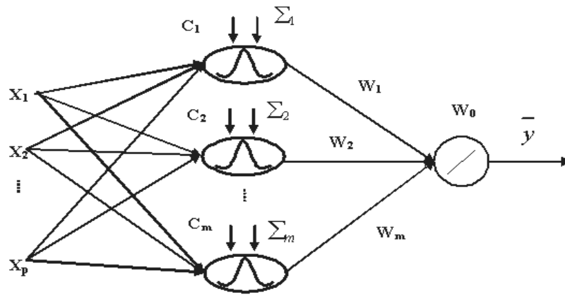
شکل ۱- ساختار کلی شبکه عصبی RBF
