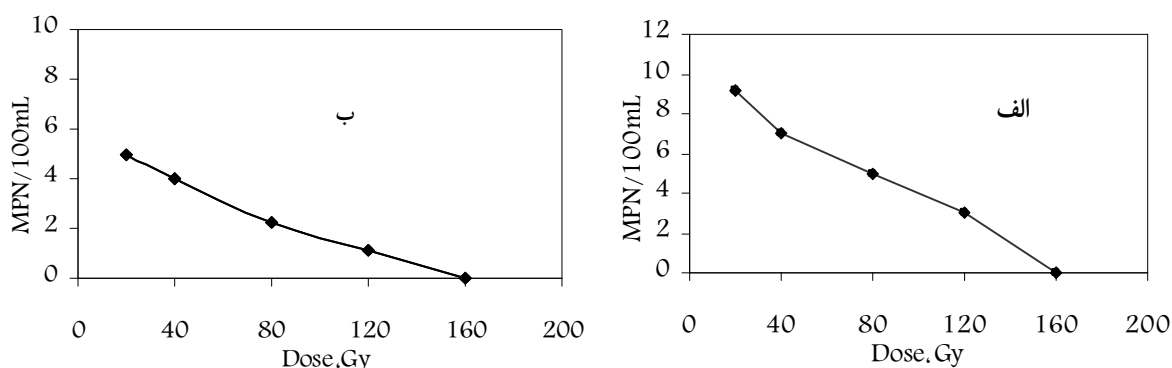
شکل ۲- نمودار میزان کلیفرم کل و مدفوعی پس از گندزدایی با اشعه گاما در دز ۱۶۰ Gy: (الف) در آب خام و (ب) در آب فیلتر شده تصفیه‌خانه آب اصفهان
