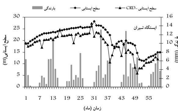
شکل ۷- رابطه بین بارندگی، سطح ایستابی اندازه‌گیری شده و سطح ایستابی شبیه‌سازی شده به روش CRD در ایستگاه تهران
