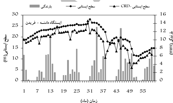
شکل ۸- رابطه بین بارندگی، سطح ایستابی اندازه‌گیری شده و سطح ایستابی شبیه‌سازی شده به روش CRD در ایستگاه دامنه فریدن
