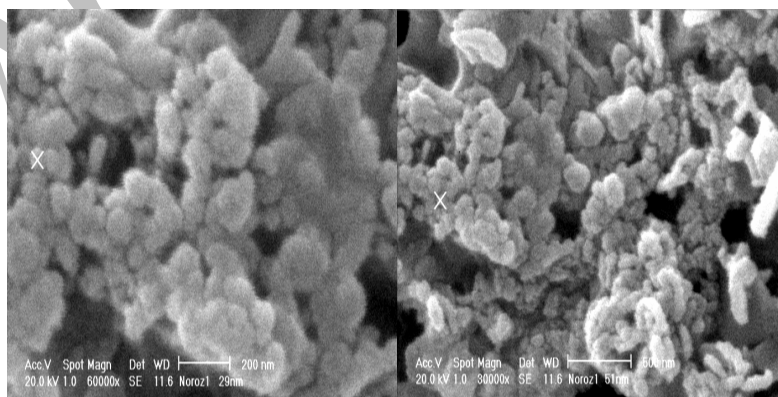
شکل ۱- تصاویر SEM از نانو ذرات آهن سنتز شده
