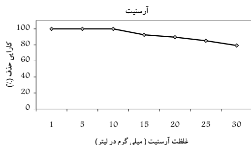
شکل ۶- بررسی تأثیر تغییرات غلظت آرسنیت و آرسنات بر کارایی حذف آن توسط نانوذرات آهن : زمان تماس ۱۰ دقیقه، 1 \text{ g L}^{-1} \text{ nZVI-C} و \text{pH}=7
