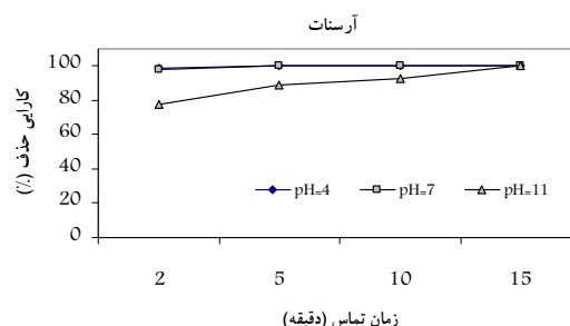
شکل ۵- بررسی تأثیر تغییرات زمان تماس و pH بر کارایی حذف آرسنیت و آرسنات 1 \text{ g L}^{-1} \text{ nZVI-C} ، غلظت آرسنیت و آرسنات 10 \text{ mg L}^{-1}
