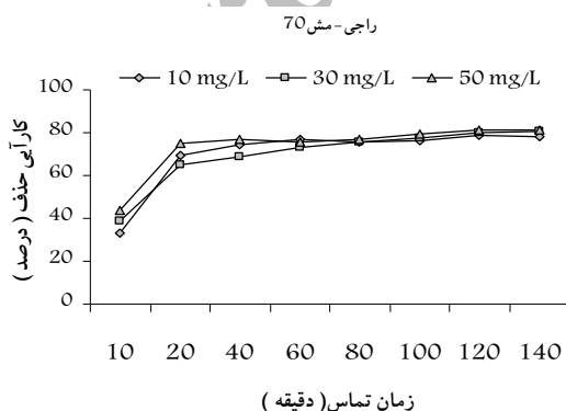
شکل ۲- نتایج حاصل از بررسی کارایی خاک اره چوب باجی در حذف سیانید از محیط‌های آبی (وزن خاک اره مورد استفاده ۵ گرم در ۵۰ میلی لیتر)
