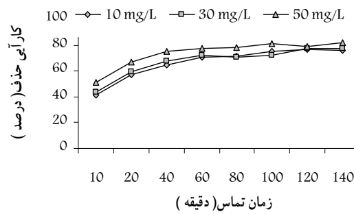
شکل ۳- نتایج حاصل از بررسی کارایی خاک اره چوب صنوبر در حذف سیانید از محیط‌های آبی (وزن خاک اره مورد استفاده ۵ گرم در ۵۰ میلی لیتر)
