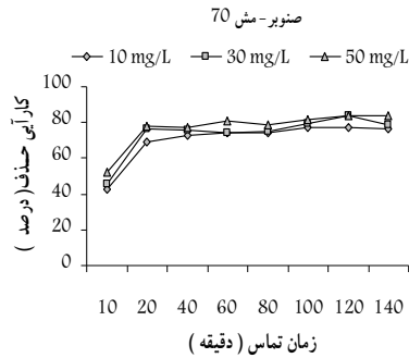
شکل ۳- نتایج حاصل از بررسی کارایی خاک اره چوب صنوبر در حذف سیانید از محیط‌های آبی (وزن خاک اره مورد استفاده ۵ گرم در ۵۰ میلی لیتر)
