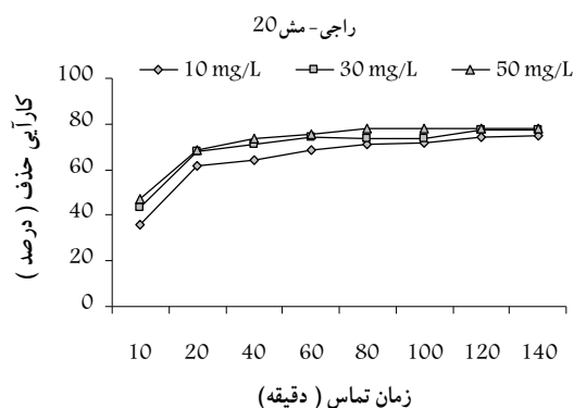
شکل ۲- نتایج حاصل از بررسی کارایی خاک اره چوب باجی در حذف سیانید از محیط‌های آبی (وزن خاک اره مورد استفاده ۵ گرم در ۵۰ میلی لیتر)
