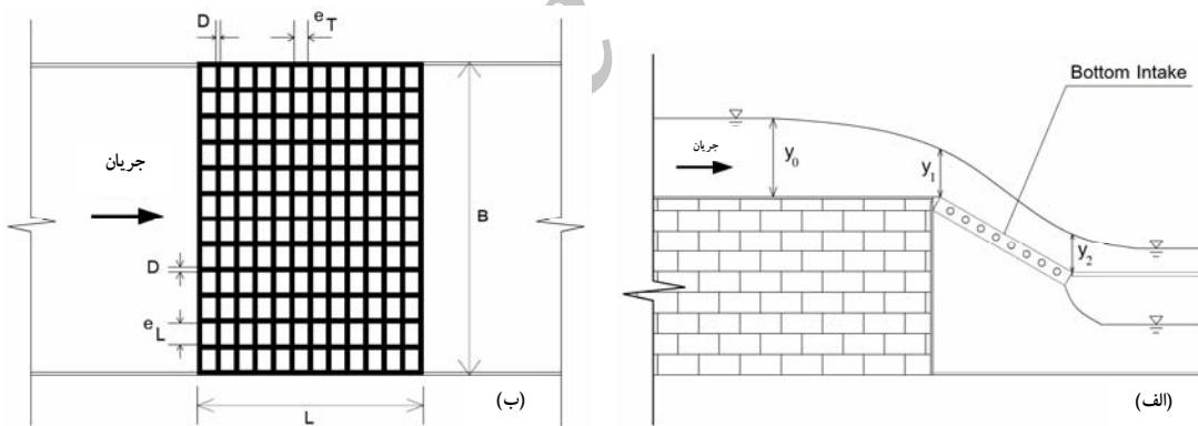
شکل ۴- الف- مقطع طولی و ب- پلان کف مشبک نصب شده داخل کانال و پارامترهای هندسی مدل
