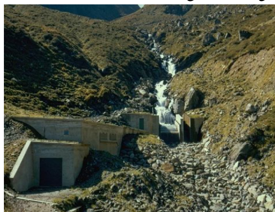
شکل ۱- آبگیری از کف برای یک نیروگاه برقابی کوچک در یک رودخانه کوهستانی [۱]
