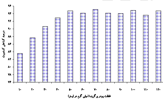
شکل ۱- درصد کاهش کدورت در غلظتهای متفاوت منعقدکننده‌ها
