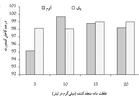
شکل ۲- درصد کاهش کدورت در حالت ترکیب منعقد کننده ها
