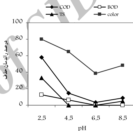
شکل ۳- بررسی تأثیر تغییرات pH بر کارایی حذف COD، BOD 5 ، TS و رنگ شیرابه محل دفن زباله شهر همدان (زمان واکنش = ۱۰ دقیقه، غلظت نانولوله کربنی = ۲/۵ گرم در لیتر)
