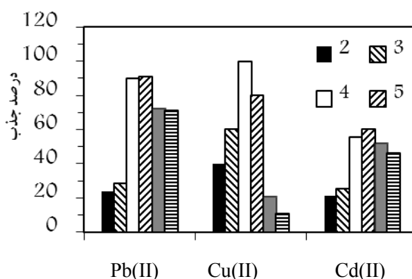
شکل ۷- اثر pH بر ظرفیت جذب تعادلی فلزات سرب، مس و کادمیم بر روی جاذب \text{NH}_2(8\text{mM})\text{-SBA-15}
