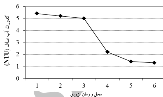
شکل ۱- تأثیر محل و زمان تزریق مگنافلاک و کلروفریک (کدورت آب خام ۵۰ NTU و pH اولیه برابر ۷)
