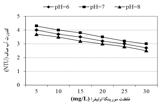
شکل ۴- تأثیر pH های مختلف بر کارایی مورینگا اولیفر با کدورت آب خام ورودی ۱۰۰ NTU (غلظت کلروفریک ۱۰ mg/l)
