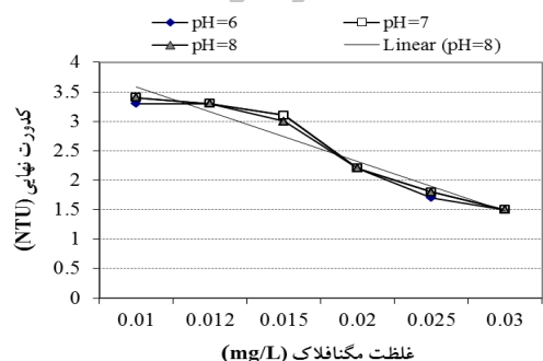
شکل ۵- نمودار کارایی مگنافلاک LT25 با کدورت آب خام ۱۰۰ NTU (غلظت کلروفریک ۱۰ mg/L)
