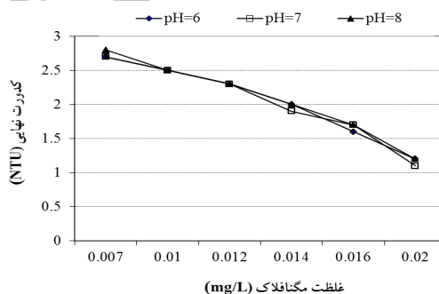
شکل ۷- کارایی مگنا فلاک LT25 در pH های مختلف با کدورت آب خام ۲۰ NTU (غلظت کلروفریک ۰/۰۱۶ mg/L)
