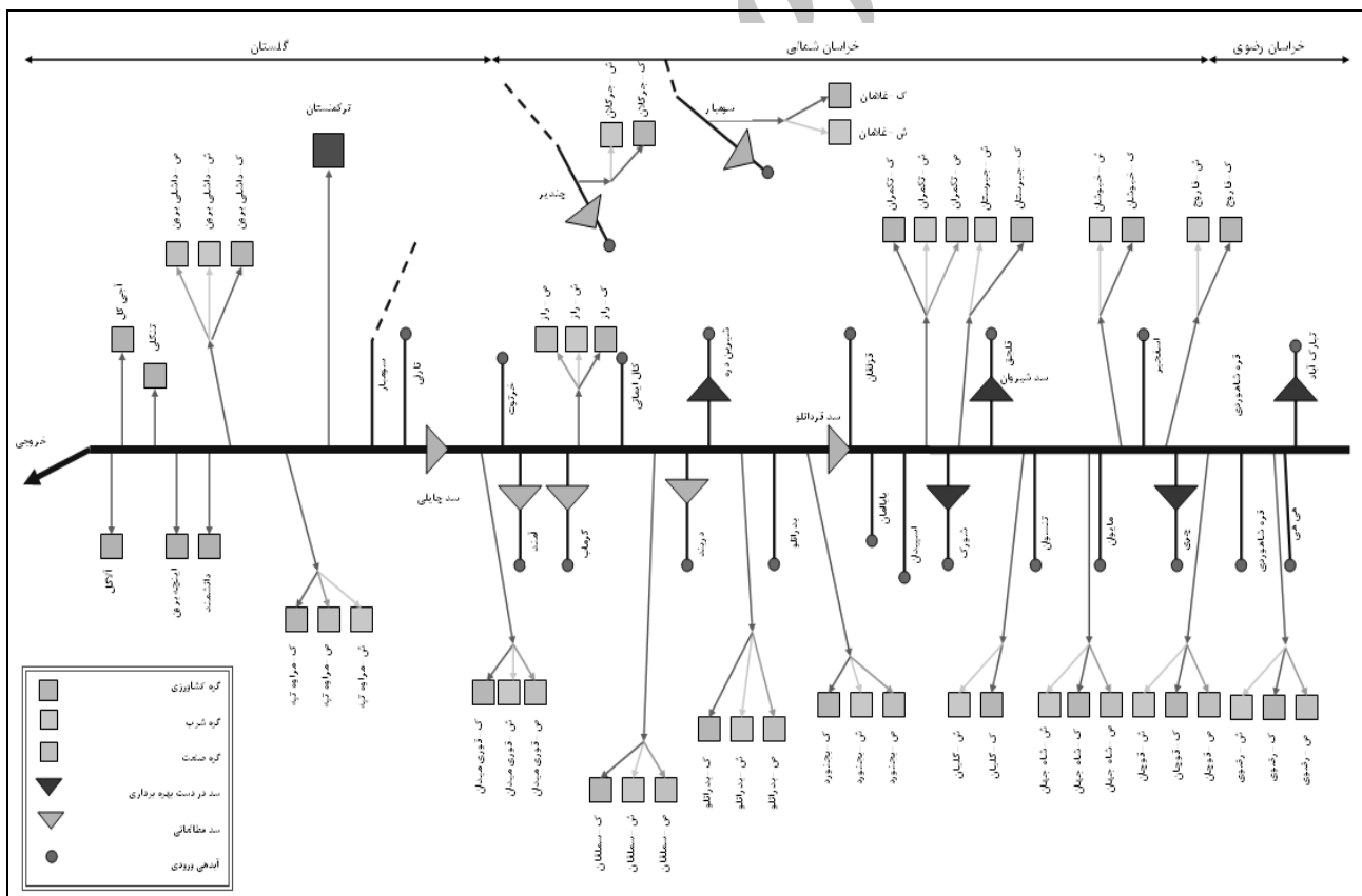
شکل ۱- توپولوژی شبکه حوضه آبریز رودخانه اترک [۲۱]
