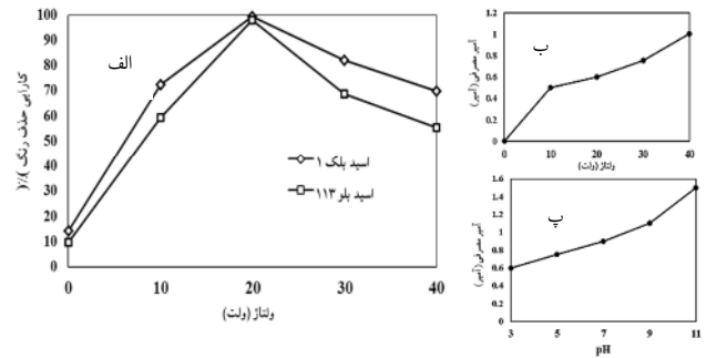
شکل ۴- الف) تأثیر ولتاژ اعمال شده در کارایی فرایند الکتروفنتون (ب) تأثیر تغییرات ولتاژ بر آمپر مصرفی (پ) تأثیر تغییرات pH در آمپر مصرفی
