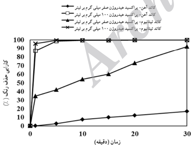
شکل ۷- تأثیر جنس کاتد و زمان ماند در کارایی فرایند الکتروفتون در حذف اسید بلک ۱
