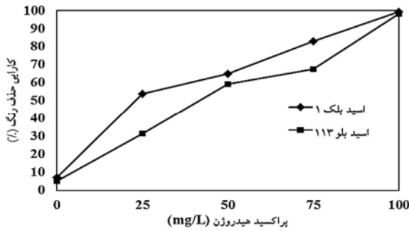
شکل ۵- تأثیر پراکسید هیدروژن در کارایی فرایند الکتروفنتون (غلظت رنگ ۱۰۰ mg/L و غلظت سدیم سولفات ۱۰۰ mg/L، pH برابر ۳، ولتاژ ۲۰ ولت، الکتروکاتد آهن)
