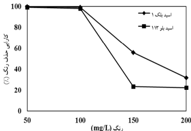
شکل ۶- تأثیر غلظت رنگ در کارایی فرایند الکتروفتون
