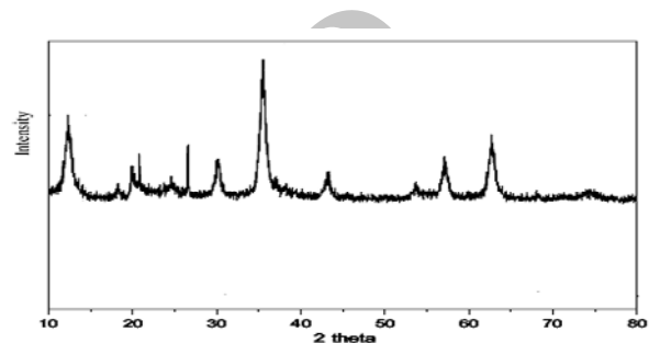
Fig. 5. XRD pattern of M-HNT/GO nanocomposite شکل ۵- طیف XRD نانوکامپوزیت M-HNT/GO
