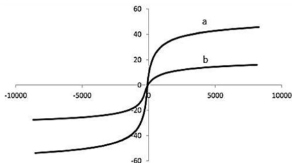
Fig. 7. VSM plot of a) Fe_3O_4 , b) M-HNT/GO شکل ۷- نمودار VSM گرفته شده از a) Fe_3O_4 - b) M-HNT/GO
