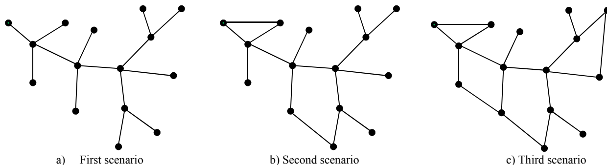
Fig. 4. Three different scenarios used for the evaluation of the reliability of water distribution network shown in Figure 3 شکل ۴- سه سناریوی مختلف به منظور ارزیابی قابلیت اعتماد شبکه توزیع آب شکل ۳
