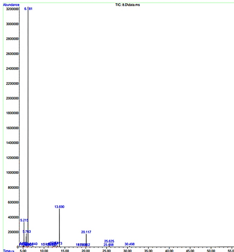
Fig. 6. GC-MS Chromatogram of the wastewater sample exposed to ultraviolet with Bi 2 O 3 nanoparticle شکل ۶- کروماتوگرام GC-MS نمونه پساب تحت تاثیر تابش UV
