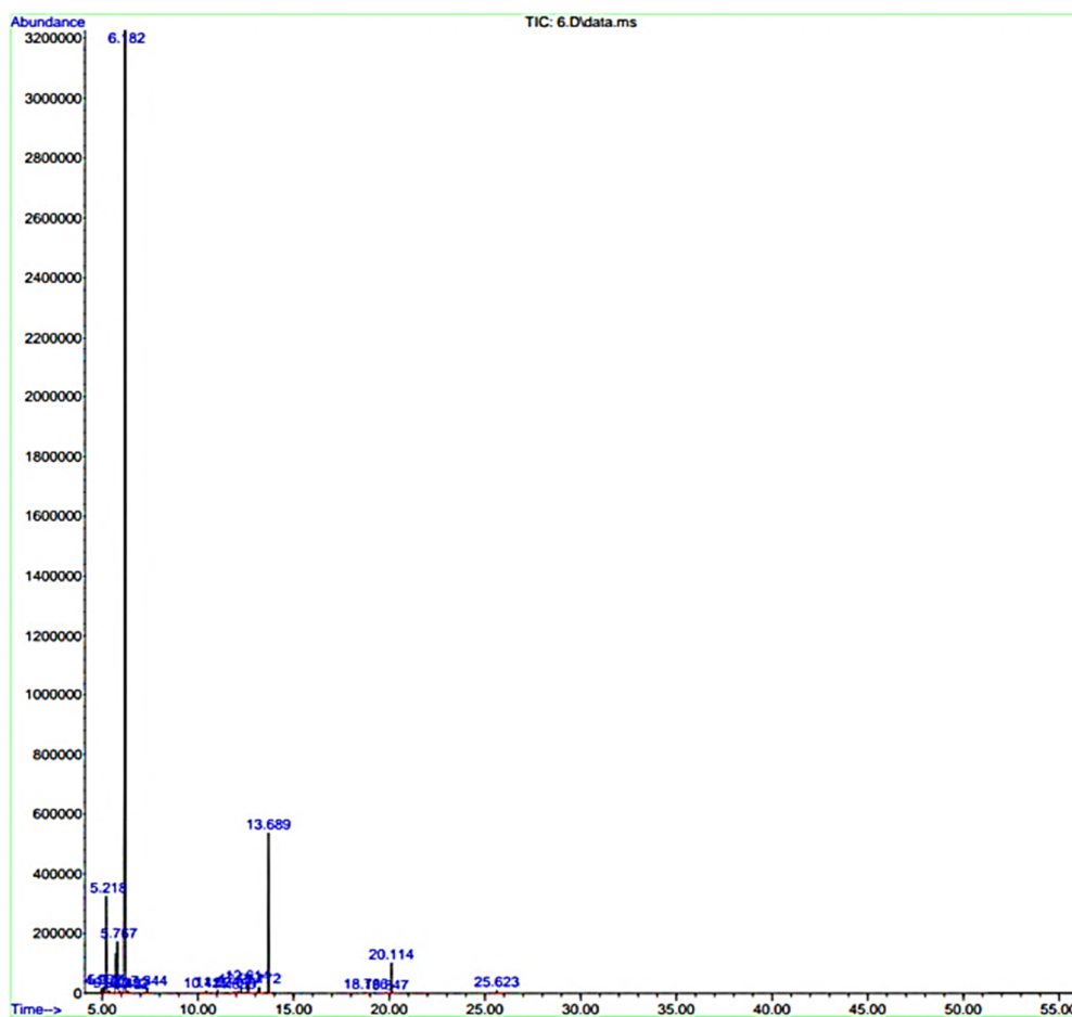
Fig. 8. GC-MS chromatogram of the wastewater sample exposed to ultrasound with Bi 2 O 3 nanoparticle شکل ۸- کروماتوگرام GC-MS نمونه پساب تحت تاثیر امواج التراسونیک و نانوذرات Bi 2 O 3
