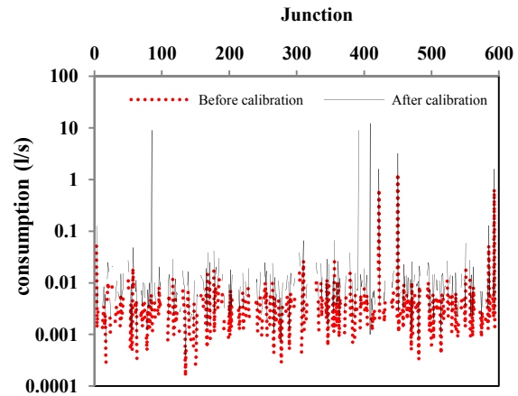
Fig. 2. Nodal demand before and after calibration شکل ۲- مصرف گره‌ای قبل و بعد از کالیبراسیون
