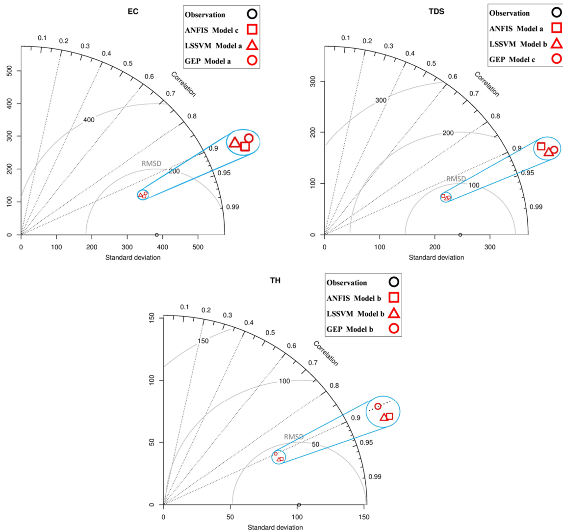
Fig. 3. Comparison between results of GEP, LS-SVM and ANFIS methods by the Taylor diagram شکل ۳- مقایسه بین نتایج روش‌های ANFIS و GEP, LS-SVM به وسیله دیاگرام تیلور
