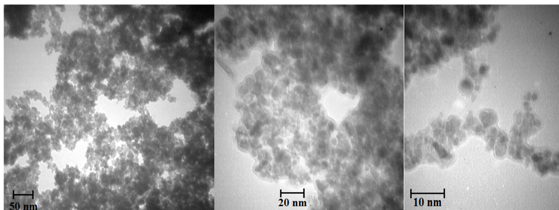
Fig. 3. The TEM image of Fe_3O_4 particles شکل ۳ - تصویر TEM مربوط به ذرات Fe_3O_4
