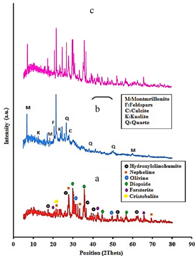
Fig. 5. XRD pattern a) natural pumice aggregate, b) bentonite nanoparticles, c) Pumice aggregate coated by bentonite nanoparticles شکل ۵- الگوی XRD (a) نانو ذرات بنتونیت، (b) سنگدانه پامیس طبیعی، (c) سنگدانه پامیس پوشش داده شده توسط نانو ذرات بنتونیت
