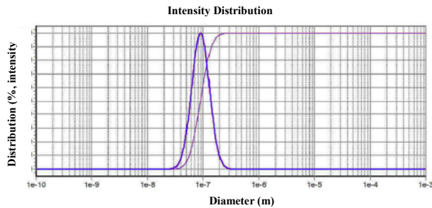
Fig. 1. Particle size analysis for bentonite شکل ۱- نمودار توزیع اندازه ذرات بنتونیت
