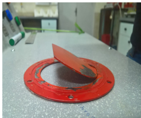
Fig. 3. Flow guide vane شکل ۳- صفحه هدایت‌کننده جریان
