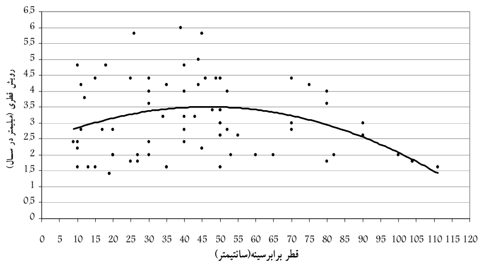
شکل 5- منحنی بررسی روند ارتباط رویش قطری بر اساس طبقات قطری
