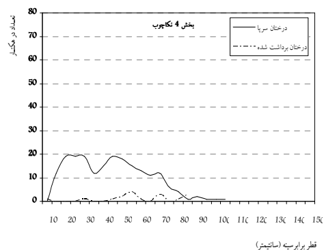
شکل 2- فراوانی درختان سریا و برداشت شده در طبقات قطر برابرسینه در سریهای 3 و 4 تیرانکلی میانشه، بخشهای 4 و 7 نکاجوب و مناطق دارابکلا و هفت‌خال از راشتانهای منطقه نکا- ظالمرو
