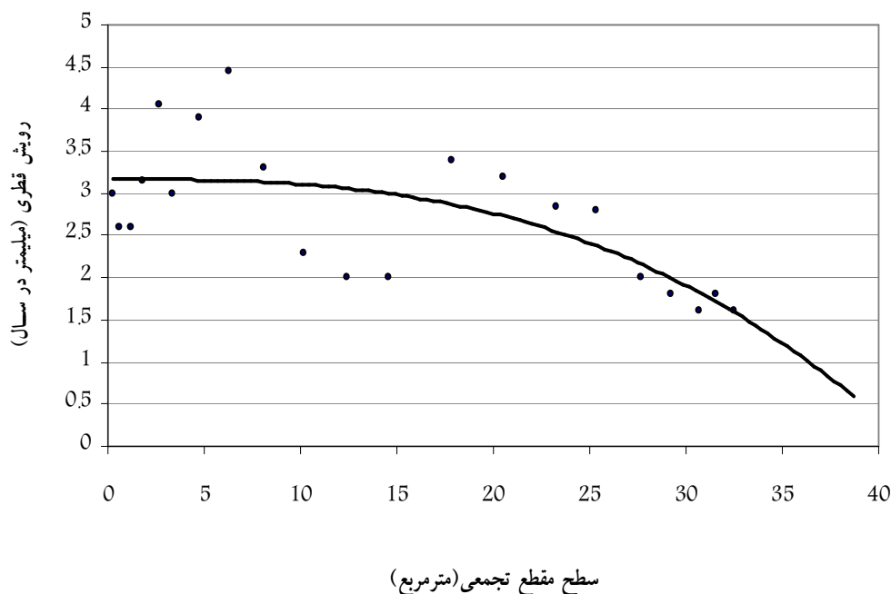
شکل 6- منحنی بررسی روند ارتباط رویش قطری سالیانه و سطح مقطع تجمعی
