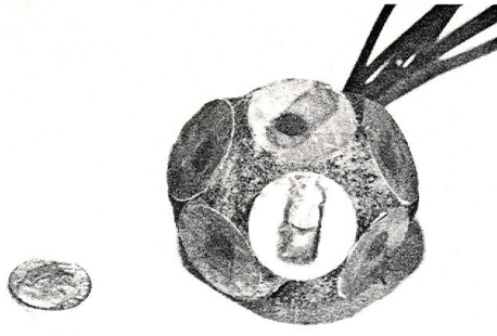
شکل 6-ب- مبدل اندازه‌گیری تنش در شش جهت
