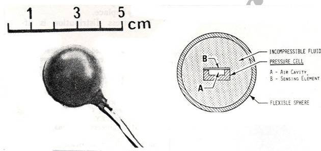
شکل 5- مبدل انعطاف‌پذیر برای اندازه‌گیری فشار هیدرواستاتیک (Verma et al. , 1976)
