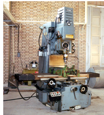
شکل 14- ماشین فرز
