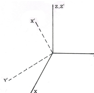
شکل 7- وضعیت محورهای X'Y'Z' نسبت به محور XYZ پس از دوران آن حول محور Z به اندازه 225°
