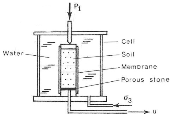
شکل 19- دستگاه آزمایش سه محوری (Mckyes, 1985)
