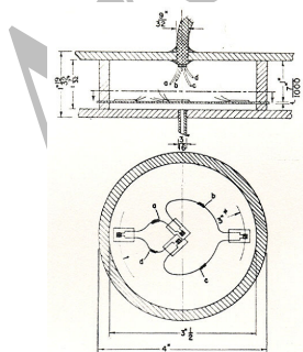
شکل 3- مبدل اندازه‌گیری تغییرات دینامیکی حجم خاک (Hovansion & Buchele, 1959)
