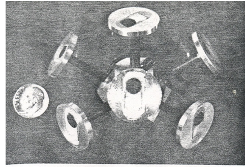
شکل 6-الف- هسته فلزی مبدل اندازه‌گیری تنش در شش جهت
