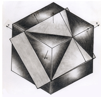
شکل 12-الف- مکعب روشن 225^\circ حول محور Z و 45^\circ حول محور X چرخیده است.
