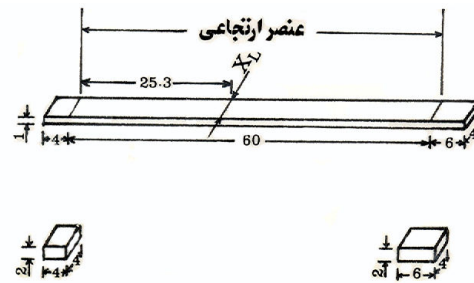
شکل 17- ابعاد عنصر ارتجاعی و پایه‌ها و محل نصب کرنش‌سنج
