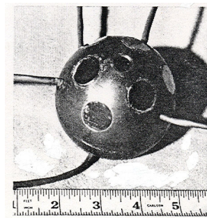
شکل 4- مبدل اندازه‌گیری تنش در شش جهت (Harris et al. , 1964)
