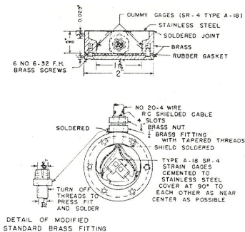
شکل 1- مبدل اندازه‌گیری فشار عمودی (Cooper et al., 1957)
