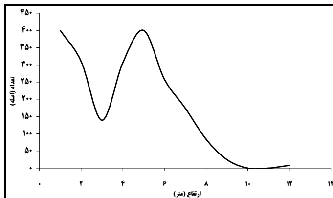
شکل ۴- نمودار پراکنش تعداد در طبقات ارتفاعی در ذخیره گاه جنگلی بلوط سرسختی
