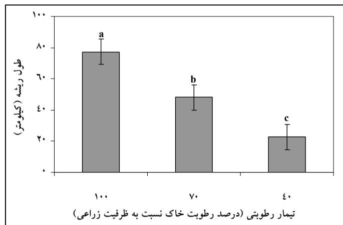
شکل ۲- تأثیر سه تیمار رطوبتی خاک بر طول ریشه اکالیپتوس سه ساله
