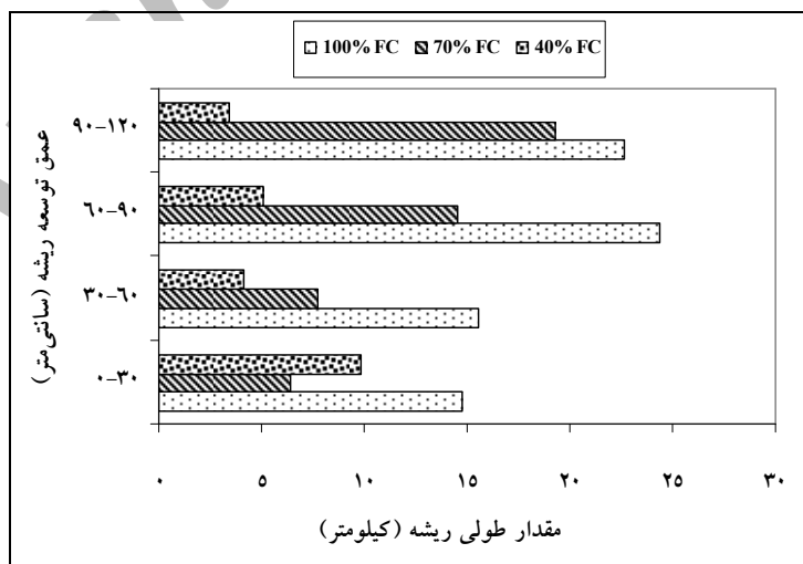
شکل ۸- مقایسه میزان طولی ریشه اکالیپتوس در اعماق مختلف خاک مربوط به هر یک از تیمارهای رطوبتی در شرایط لایسیمتری (FC: ظرفیت زراعی)
