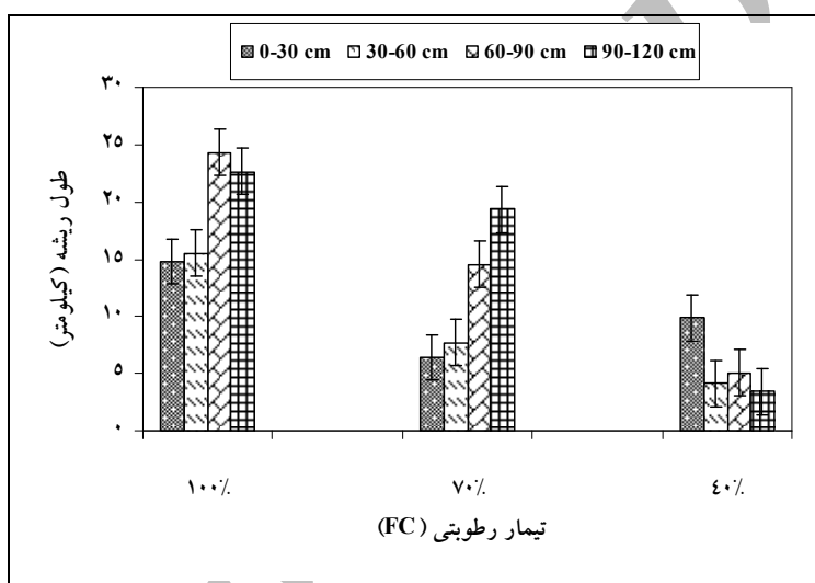
شکل ۷- پراکنش طولی ریشه اکالیپتوس در اعماق مختلف خاک در سه تیمار رطوبتی در شرایط لایسیمتری (FC: ظرفیت زراعی)
