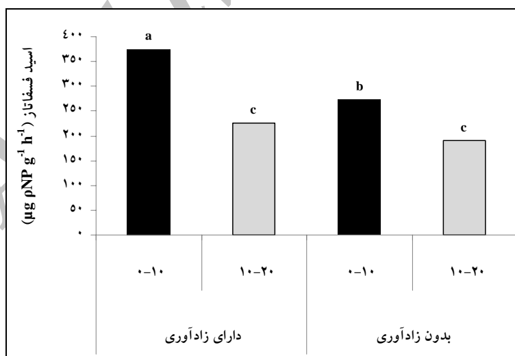
شکل ۱- فعالیت آنزیم اسید فسفاتاز در عمق‌های مختلف خاک دارای زادآوری و بدون زادآوری (حروف مختلف نشان دهنده تفاوت سطوح معنی‌دار هستند)
