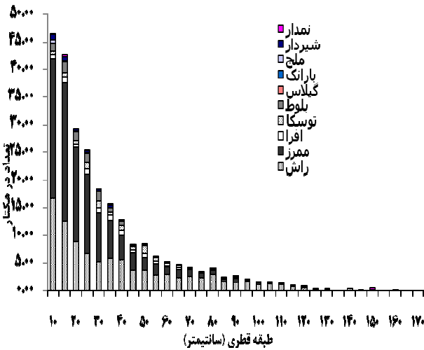
شکل ۹- منحنی پراکنش تعداد در طبقات قطری کل گونه‌ها در کل بخش گرازبن در سال ۸۲
