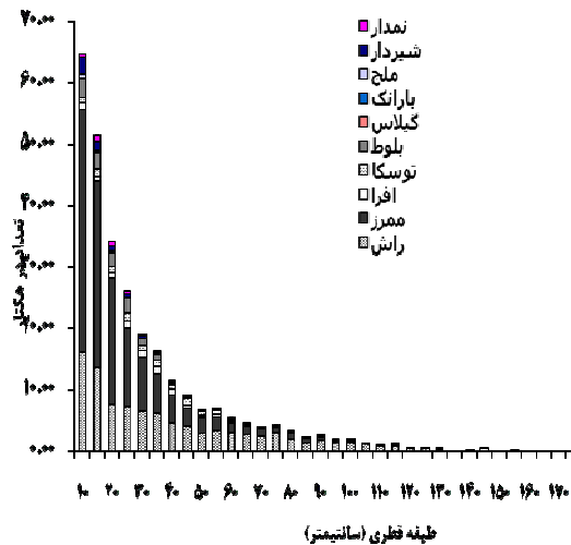
شکل ۸- منحنی پراکنش تعداد در طبقات قطری کل گونه‌ها در کل بخش گرازبن در سال ۹۱
