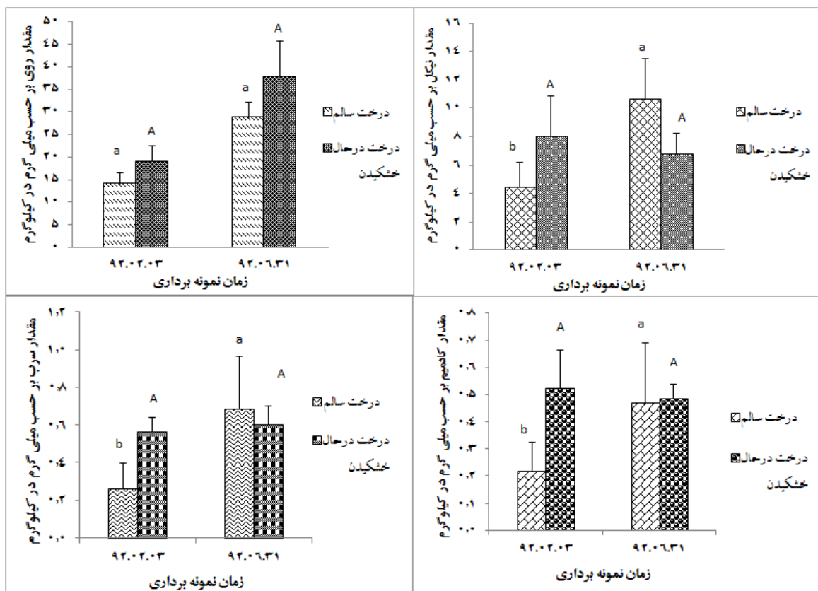
شکل ۶- مقدار چهار عنصر جذب شده در شاخه‌های درخت برودار در دوره شش‌ماهه بهار و تابستان ۱۳۹۲ (حروف نامشابه بزرگ نشانگر معنی‌داری بودن اختلاف میانگین‌ها در درختان رو به خشکیدن و حروف نامشابه کوچک نشانگر معنی‌داری بودن اختلاف میانگین‌ها در درختان سالم هستند).
