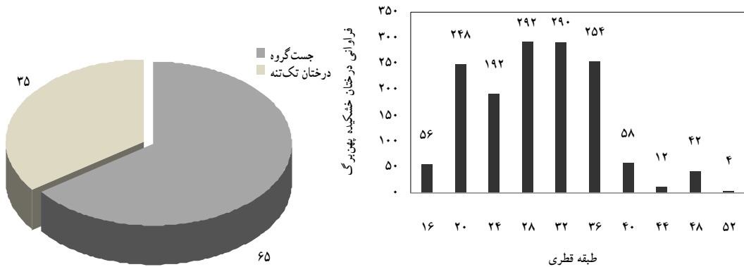
شکل ۳- فراوانی درختان خشکیده پهن برگ برحسب طبقه‌های قطری
