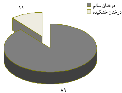
شکل ۱- فراوانی (درصد) پایه‌های سالم و خشکیده
