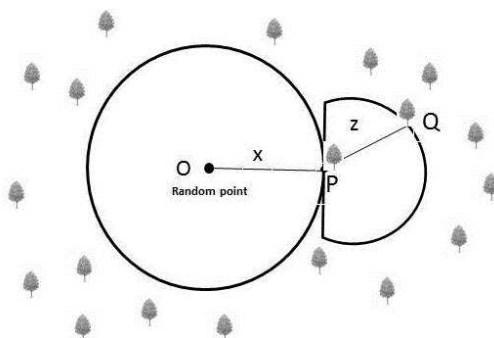
شکل ۲- نمای شماتیک نمونه‌گیری مربع T: فاصله X بین نقطه تصادفی O و نزدیک‌ترین موجود زنده (P) و فاصله Z بین فرد (P) و نزدیک‌ترین همسایه یعنی Q. در انتخاب Q افرادی که در همان طرف نیم‌صفحه قرار می‌گیرند (مثل O)، در نظر گرفته نمی‌شوند (Krebs, 1999).
