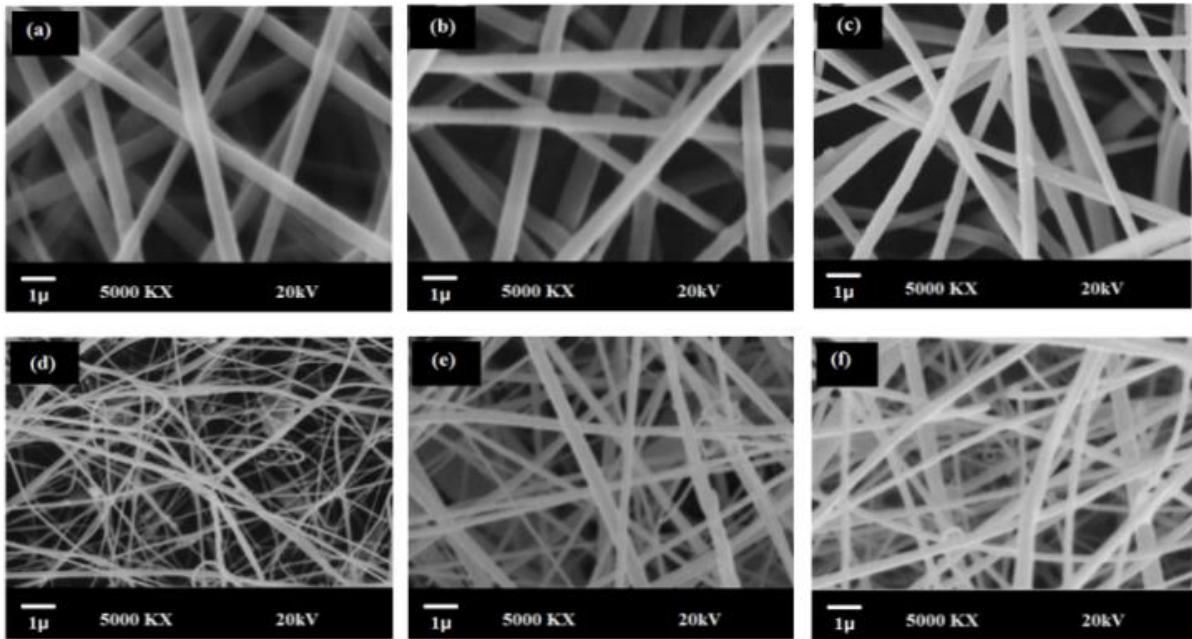
شکل ۲- تصاویر SEM نمونه‌های نانوالیاف در فاصله‌های مختلف بین نوک سوزن تا جمع‌کننده: (a) نانوالیاف TiO_2 (b) نانوالیاف CoFe_2O_4 (c) نانوالیاف TiO_2/CoFe_2O_4 و (d) نانوالیاف TiO_2 (e) نانوالیاف CoFe_2O_4 (f) نانوالیاف TiO_2/CoFe_2O_4
