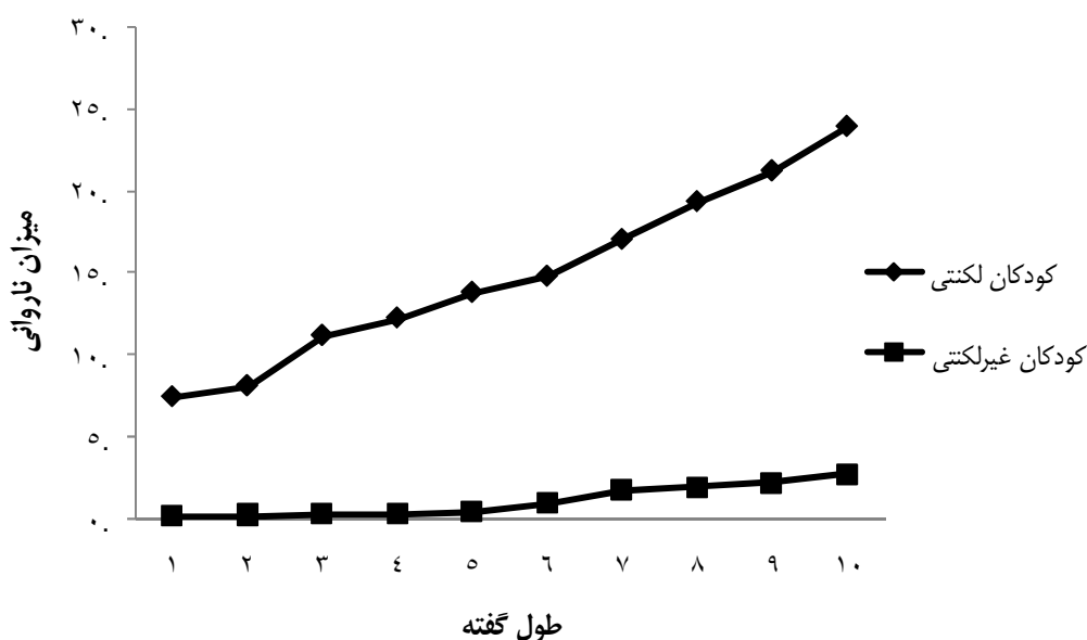
نمودار ۱- میزان ناروانی بر حسب افزایش طول گفته در ده دسته جمله در دو گروه کودک لکتی و غیرلکتی فارسی زبان
