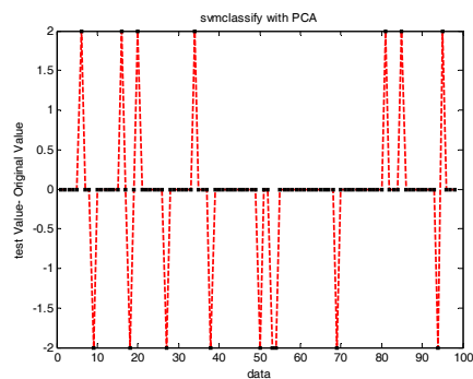
شکل ۱۰- نتیجه تست داده‌ها با انتخاب ۱۰ ویژگی به روش PCA با وجود طبقه‌بند SVM
