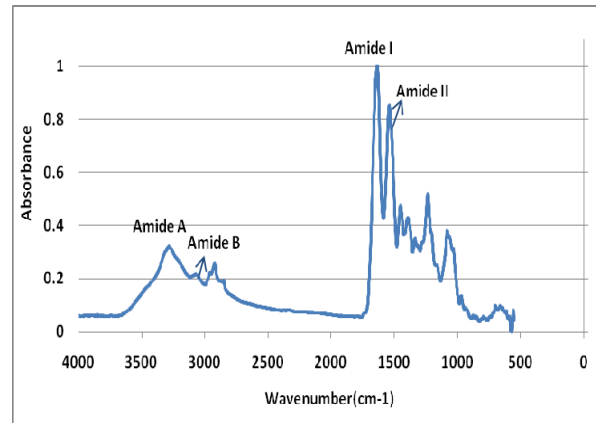
شکل ۳: طیف کلی FTIR نمونه تابش نشده
