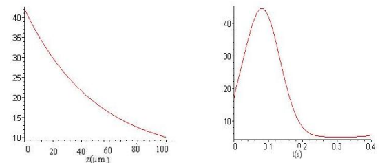
نمودار ۴ الف: تغییرات دما بر حسب عمق برای انرژی ۸ ژول
