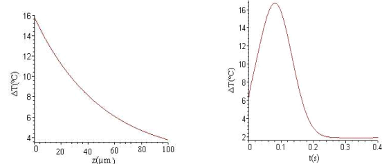
نمودار ۳ الف: تغییرات دما بر حسب عمق زمان برای انرژی ۲/۴ ژول
