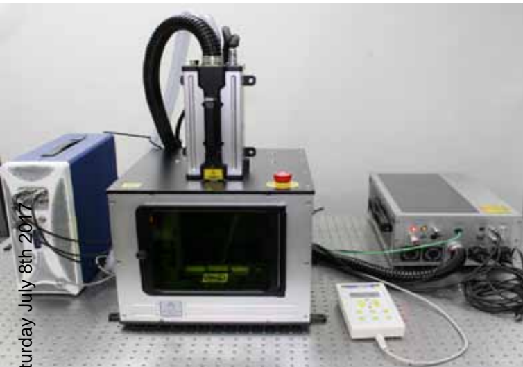
شکل ۲: سامانه LIBSCAN ۱۰۰۰
