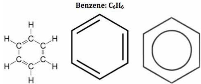
شکل ۱: ساختار مولکولی بنزن
