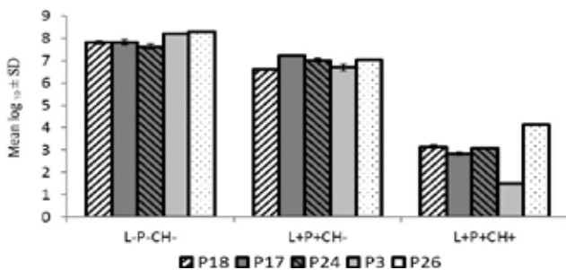
نمودار ۲: تعداد سلول های زنده در بیوفیلیم جدایه های P. aeruginosa پس از غیرفعال سازی فتودینامیکی ضد میکروبی با متیلن بلو. غلظت نهایی متیلن بلو ۲۰۰ μM، غلظت نهایی کیتوزان ۱۰۰۰ μg/ml، دوز نوری ۴۷ J/cm ۲ . (کیتوزان: CH، حساسگر نوری: P، نور لیزر: L)
