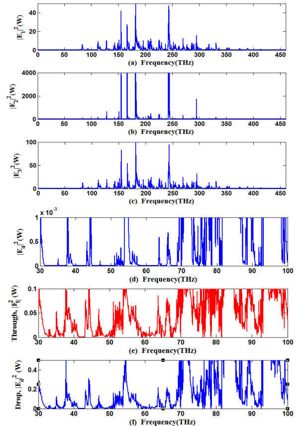
شکل ۳. نتیجه شبیه‌سازی پالس نوری که توسط سیستم PANDA در طول موج مرکزی ۱,۳ میکرومتر تولید می‌شود. جایی که (a), (b), (c), (d), (e), (f) توان خروجی داخل سیستم PANDA وجود دارد.
