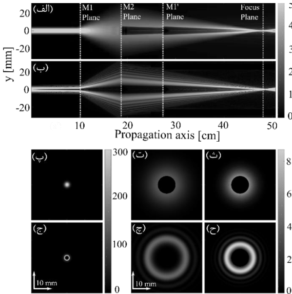
شکل ۵: توزیع شدت در صفحه xz در جهت انتشار برای (الف) باریکه گاوسی و (ب) باریکه چرخان. توزیع شدت در صفحه xy در مقاطع M_1 ، M_2 ، M_1' برای (ت)، (ث) و (ج) باریکه گاوسی و (چ)، (ج) و (خ) باریکه چرخان.
