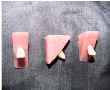
شکل ۴: دندان های مانت شده و ترمیم شده، آماده برای آزمایش شکست
