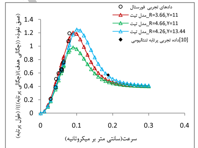
شکل ۵- منحنی‌های محاسبه شده برای Y و R پرتابه تنتالیومی.
