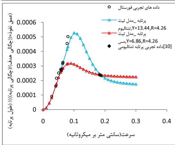
شکل ۶- محاسبه Y و R برای پرتابه‌هایی از جنس مس و تنتالیوم و هدف بتنی.
