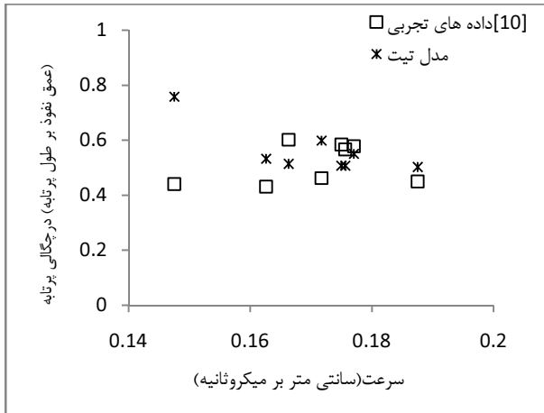
شکل ۷- مقایسه نتایج به دست آمده از مدل تحلیلی حاضر با نتایج تجربی.
