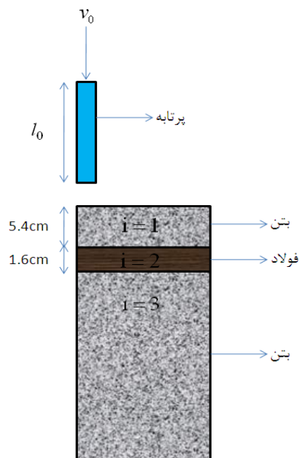
شکل ۳- هدف چند لایه بتن- فولادی.
