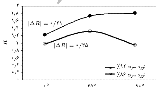
شکل ۴. مقایسه‌ی نسبت کرنش در جهات مختلف نسبت به راستای نورد برای دو نمونه با دمای پایانی نورد متفاوت (۶۰۰ و ۵۰۰) و نورد سرد شده در ۹۲ درصد، و دو مرحله تابکاری در ۴۵ درجه.
