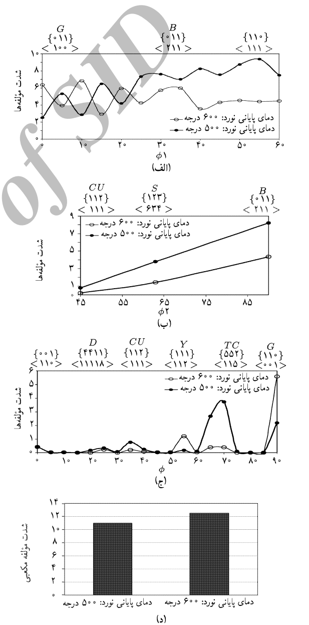
شکل ۳. چگالی مؤلفه‌های بافتی در رشته‌های: الف) \alpha ; ب) \beta ; ج) \gamma ; د) مؤلفه‌ی مکعبی برای دو نمونه با دماهای پایانی نورد متفاوت (۵۰۰ و ۶۰۰) و نورد سرد شده تا کرنش ۹۲ درصد و دومرحله تابکاری در ۴۵۰.
