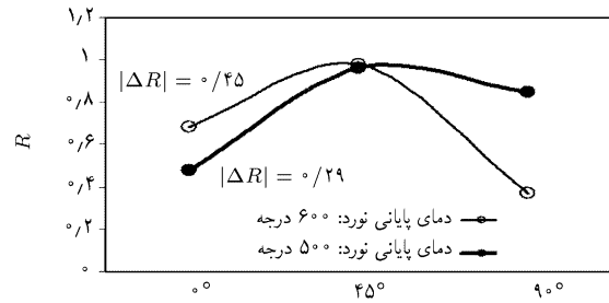
شکل ۵. مقایسه‌ی نسبت کرنش در جهات مختلف نسبت به راستای نورد برای دو نمونه با دماهای پایانی نورد متفاوت (۶۰۰ و ۵۰۰) و نورد سرد شده در ۹۲ درصد و دو مرحله تابکاری در ۴۵ درجه.
