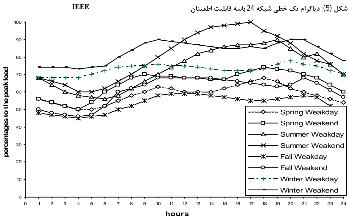
شکل (4): نمودار میانگین تقاضای روزانه نسبت به ماکزیمم بار، برای سالهای بهره برداری، نمودار بار نسبت به تغییر فصل و روزهای تعطیل و غیر تعطیل متفاوت لحاظ شده است
