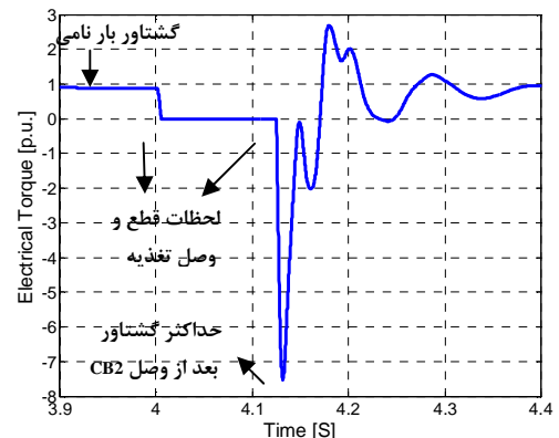
شکل (۷): گشتاور الکتریکی موتور در حالت نرمال، قطع تغذیه در ۴ ثانیه و وصل کلید CB_2 در زمان ۴,۱۲۵ ثانیه
