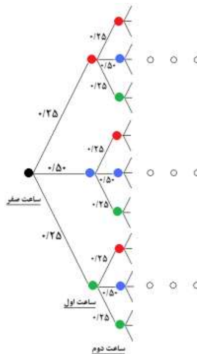
شکل (۵): درخت سناریو قیمت انرژی
