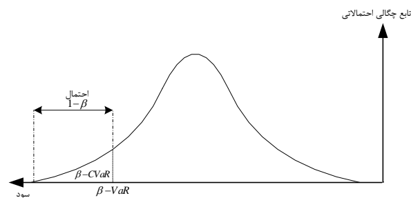
شکل (۱): مفهوم گرافیکی شاخص‌های CVaR و VaR
