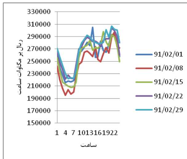
شکل (۳): منحنی تغییرات قیمت انرژی
