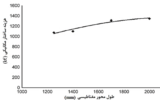
شکل (۲): نمودار تقریبی هزینه ساختاری (یورو) نسبت به طول محور مغناطیسی
